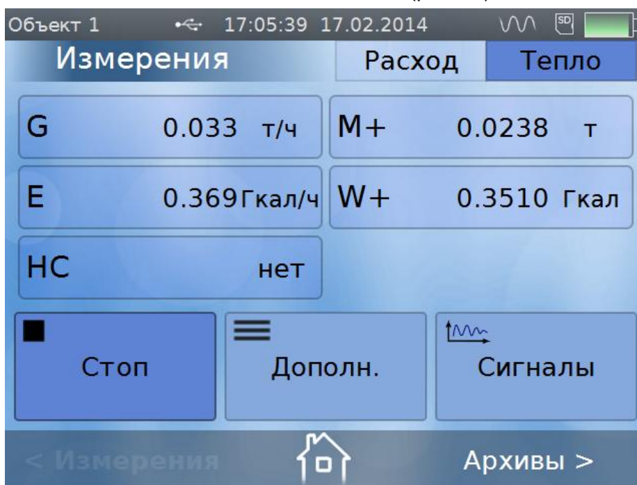
Рис.14. Окно «Измерения / Тепло»
