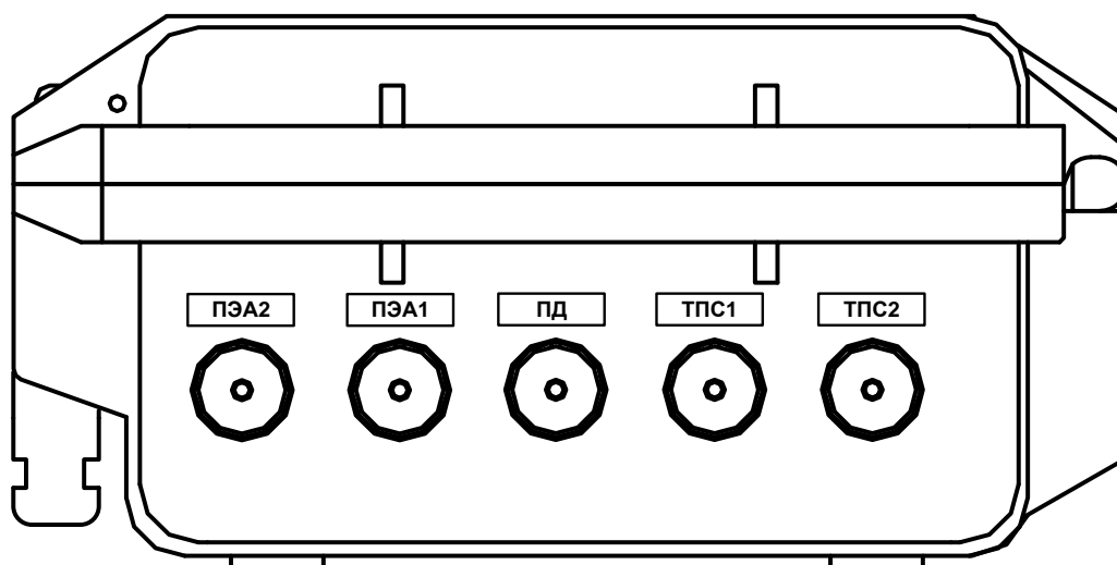
г) вид со стороны разъемов связи с ПЭА и датчиками температуры и давления
