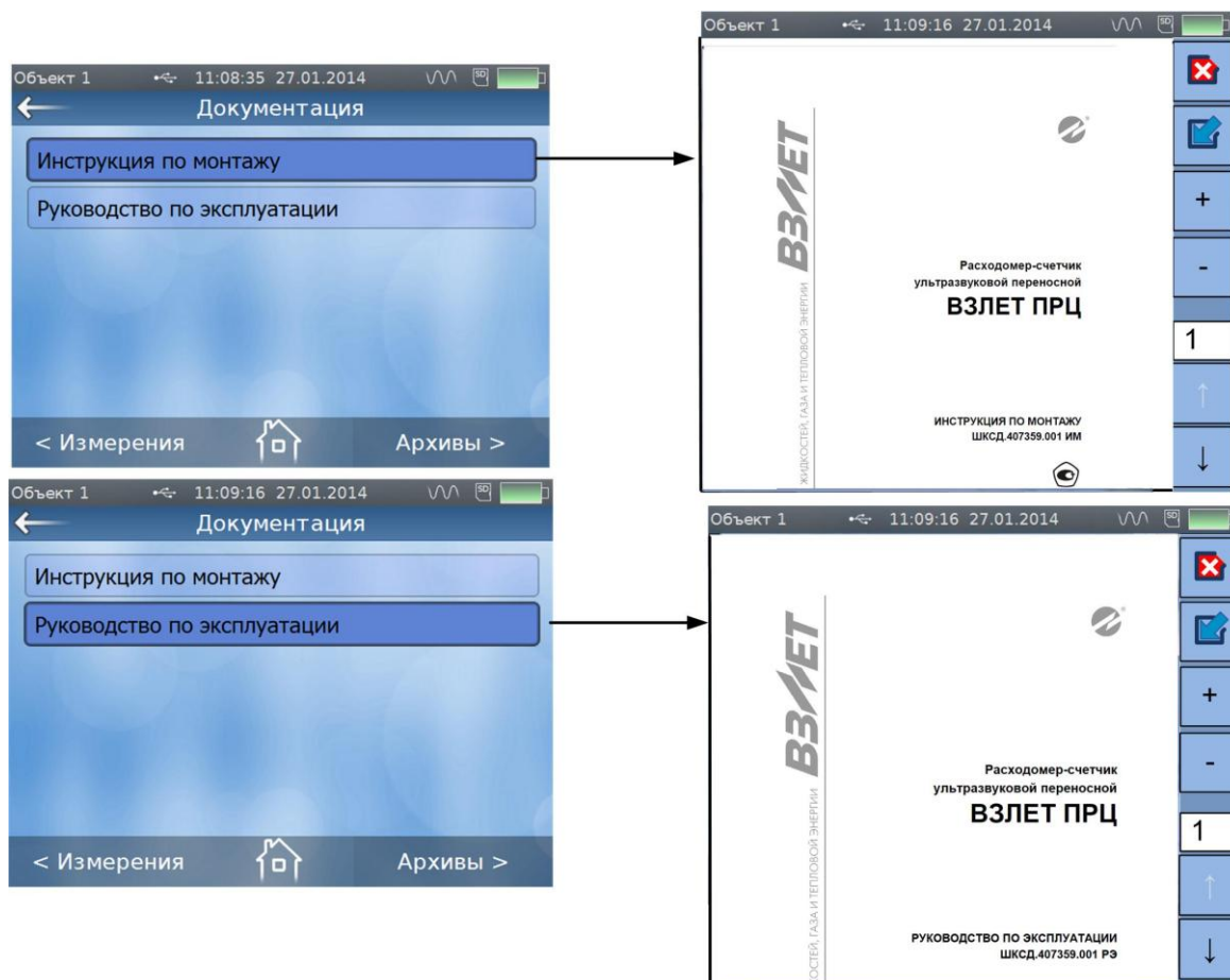
Рис.18. Окно «Документация»
