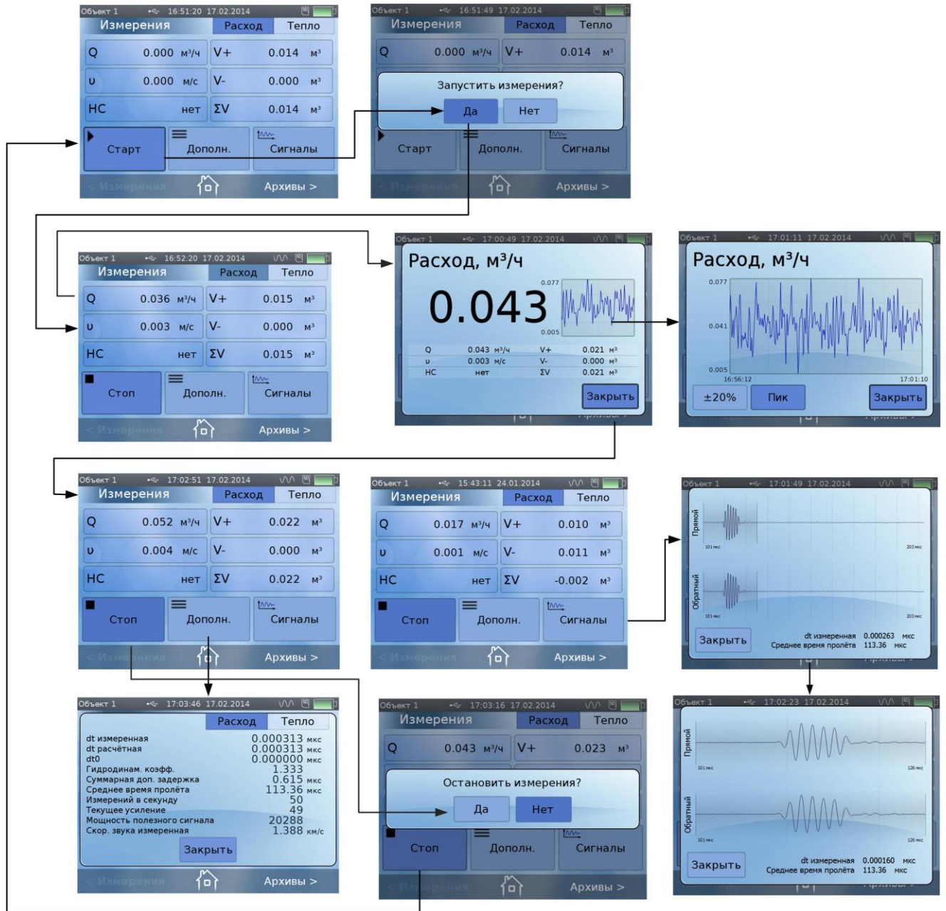
Рис.13. Окно «Измерения / Расход»
